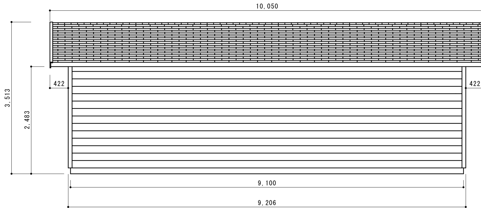
側面図
